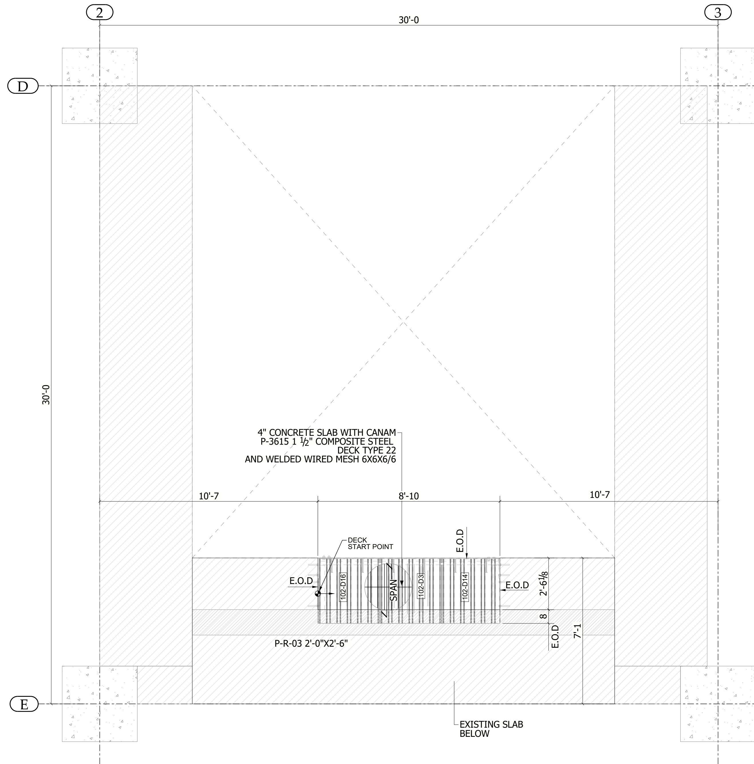
DECK PLAN @ RDC @ B/DECK EL. 146'-8 (REFER : VUE EN PLAN -PARTIELLE RDC- S2.0)
